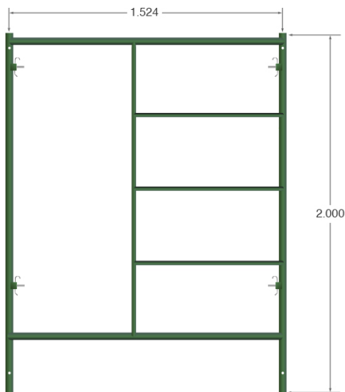
MARCO DE 2.00 Mts. MODELO: 1-156-2 PESO: 21.00 Kg
