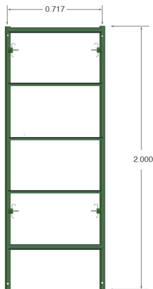
MARCO ANGOSTO MODELO: 1-156-2A PESO: 15.00 kg
