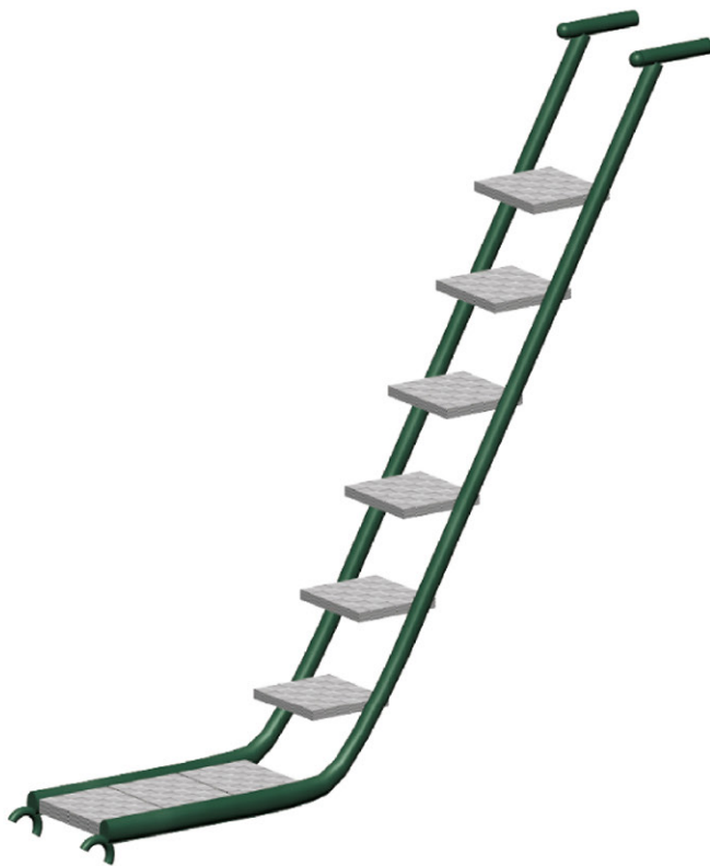
ESCALERA METALICA MODELO: 1-ESC-0 PESO: 46.00 Kg
