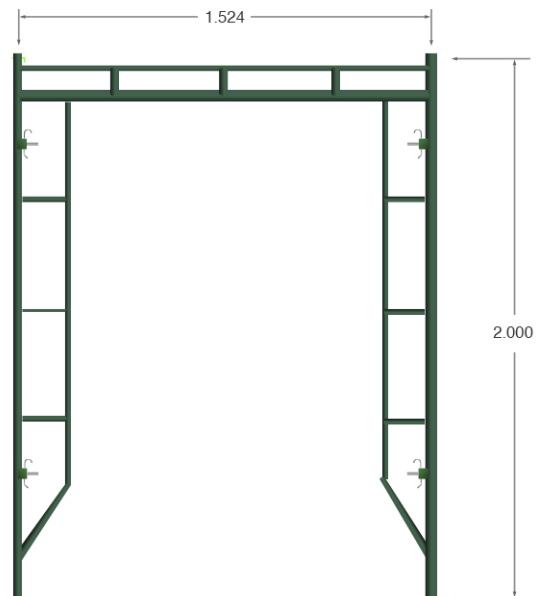
MARCO DE 2.00 Mts. PUENTE MODELO: 1-156-6 PESO: 26.60 Kg
