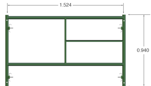
MARCO DE 0.94 Mts. MODELO: 1-153-0 PESO: 14.00 Kg
