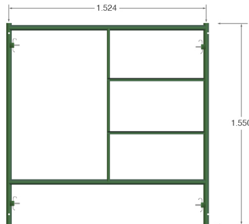
MARCO DE 1.55 Mts. MODELO: 1-155-0 PESO: 18.50 Kg
