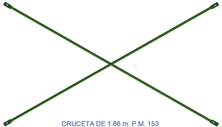
CRUCETA DE 1.86 m. P.M. 153 MODELO: 1-253-05 PESO: 4.00 Kg
